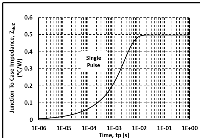
图. 25 热阻曲线
