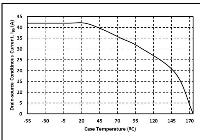
图. 23 漏端电流和温度关系曲线
